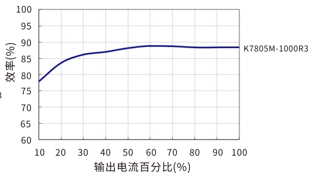
效率Vs输出负载 (标称输入)
