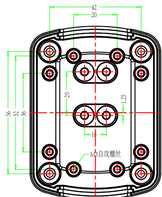
底壳内视图
