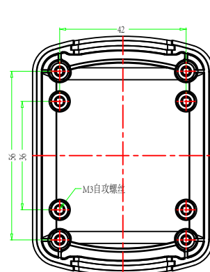
上壳内视图
