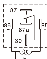
带二极管型(D2型)
