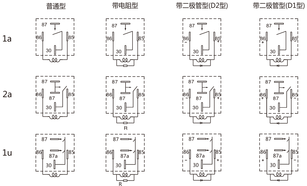
接线图 (底视图)
