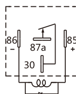
接线图 (底视图)
