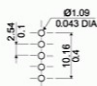
P.C.B. LAYOUT
