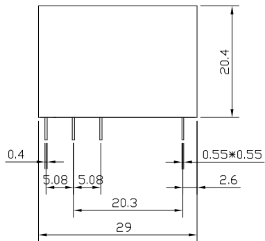
安装图
