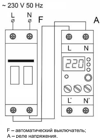
Рисунок 2 – Схема подключения
