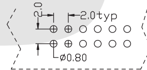
P.C.B Layout
