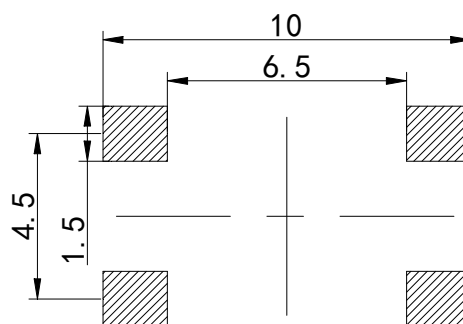
PCB焊接尺寸图
