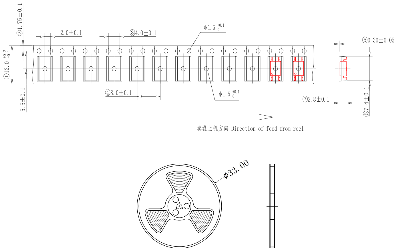
图 13 编带包装示意图
