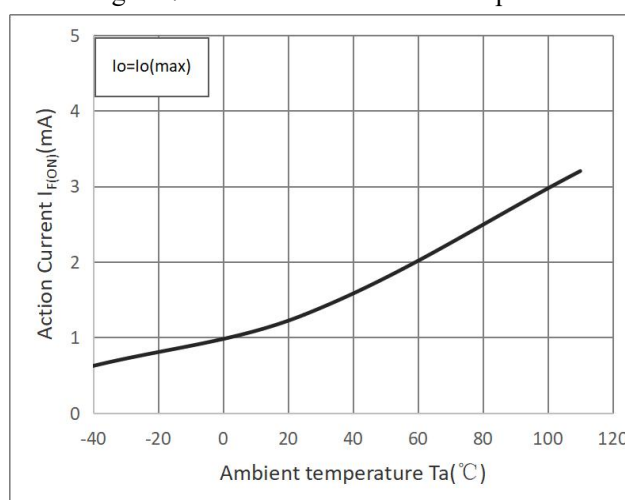
图 8 I_F(ON)-T_a 特性曲线
