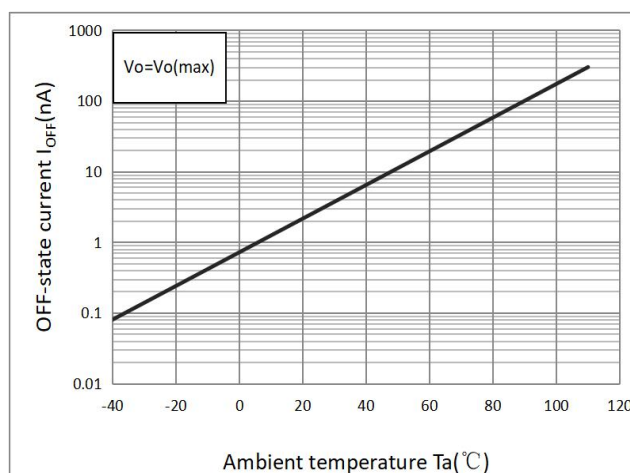
图 6 I_OFF-T_a 特性曲线
