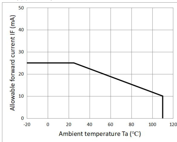
图 4 I_F - T_a 特性曲线
