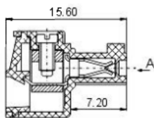
Разрез A-A
