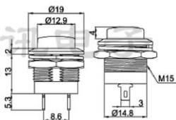
安装尺寸 (Mounting)
