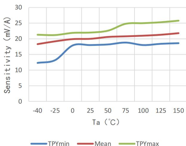
100A灵敏度随温度变化
