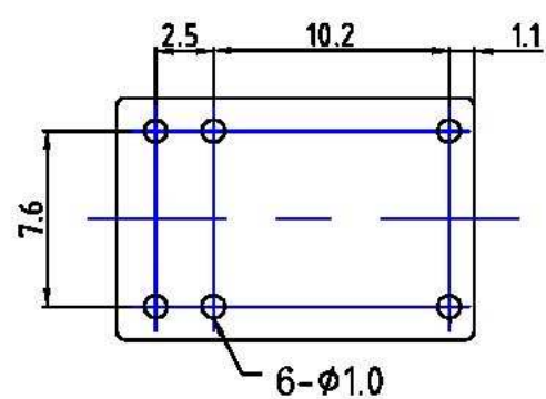
PC Board Layout 安装图
