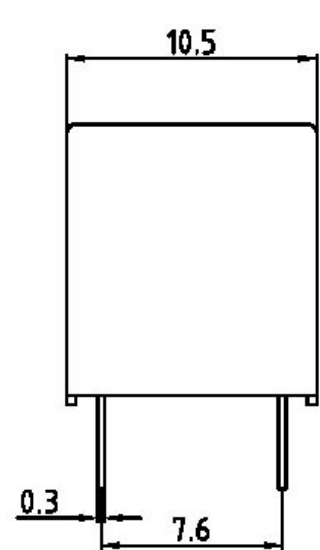
Outline Dimension (mm) 外形尺寸(mm)
