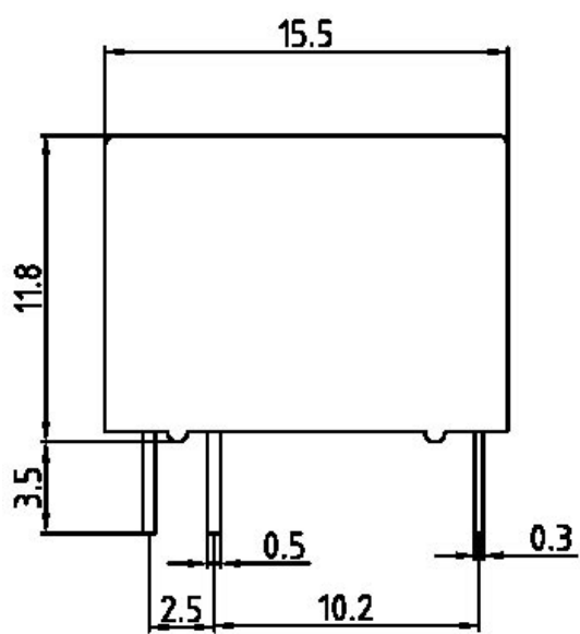
Outline Dimension (mm) 外形尺寸(mm)
