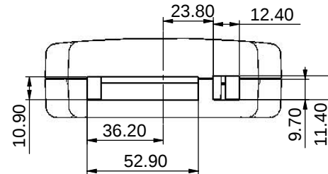
视图 D
