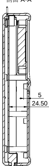
剖面 A-A
