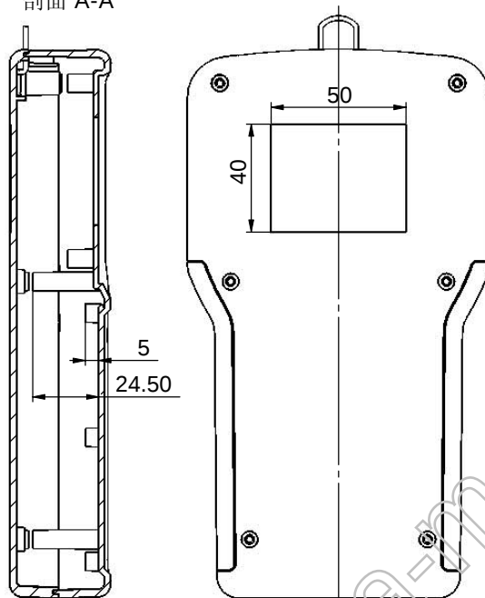
剖面 A-A
