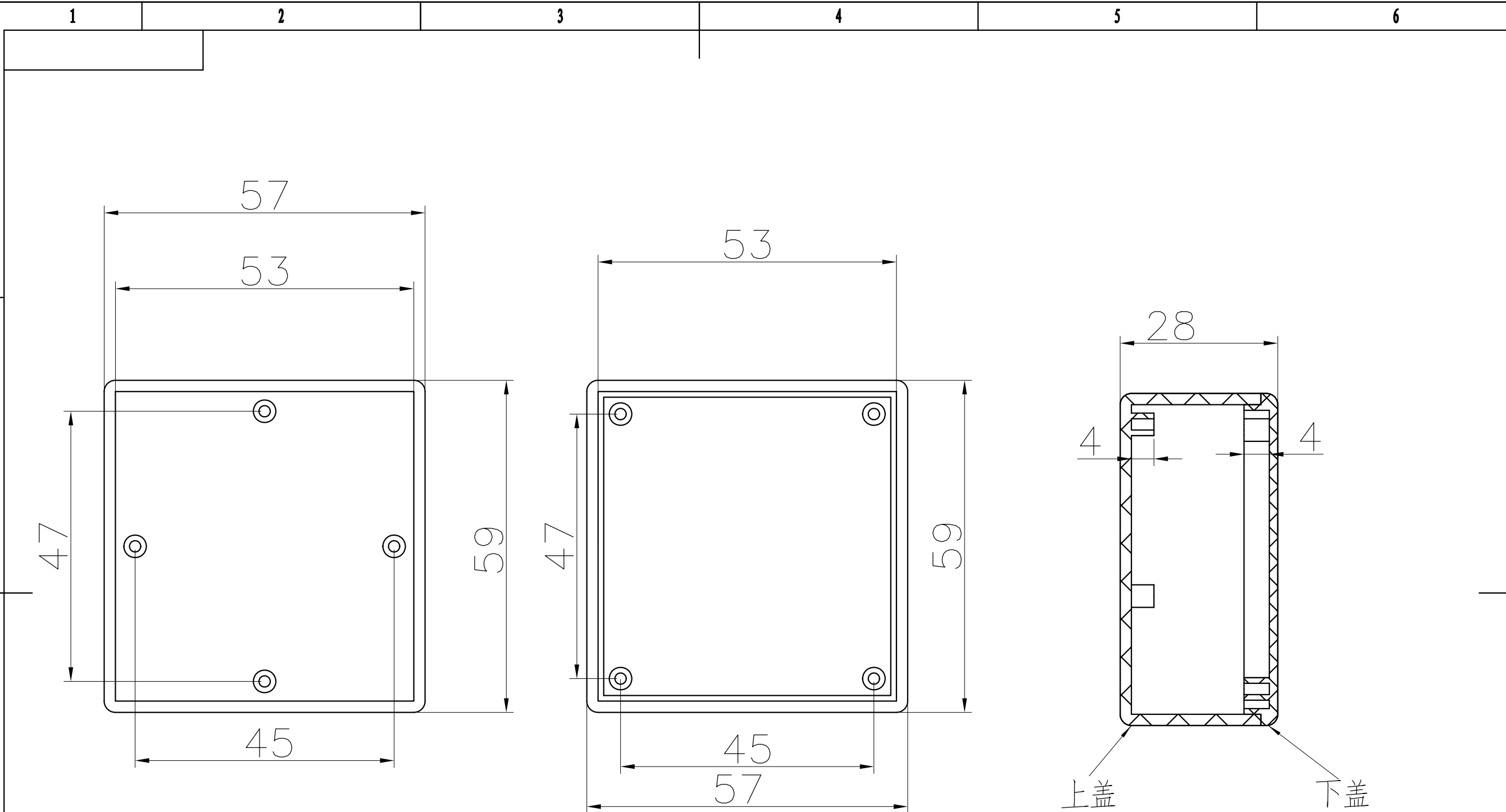
上盖底视图
