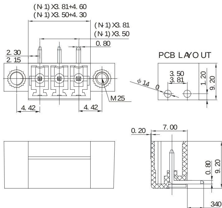
15EDGRM-3.5 15EDGRM-3.81
