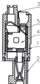
SEC A-A
