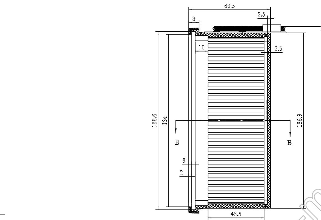
截面 A-A
