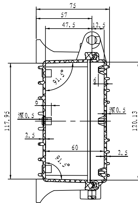
截面 A-A
