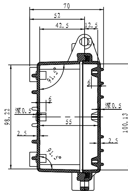
截面 A-A
