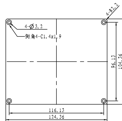
面板
