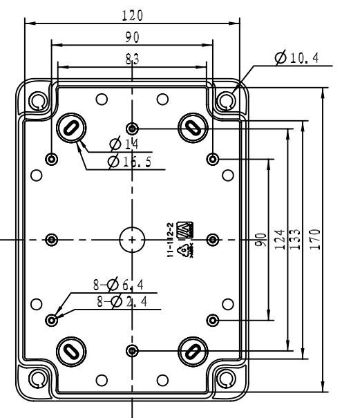
下盖正视图
