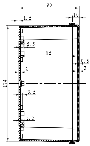
剖面 B-B
